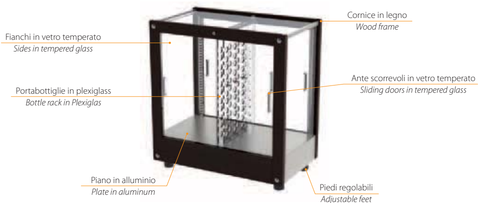
MODELLO CON ANTE SCORREVOLI SU ENTRAMBI I LATI MODEL WITH SLIDING DOORS ON BOTH SIDES
